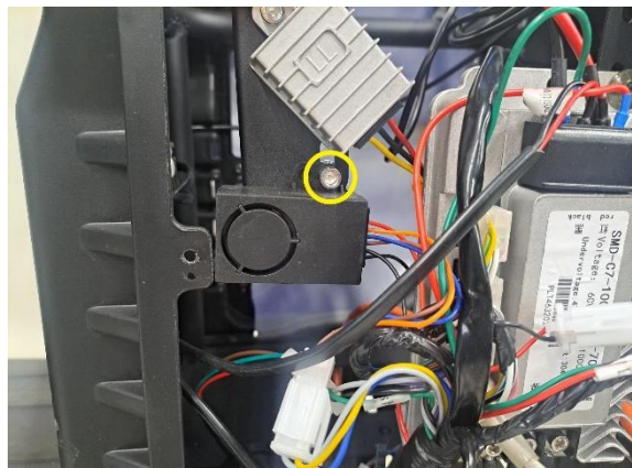
Irrota hälyttimen kiinnityspultti (kuusiokoloavain 5 mm) jolla on vastamutteri (kiintoavain 10 mm).
